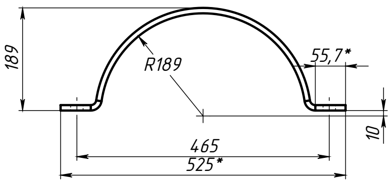
Поз.4 (Полухомут)
